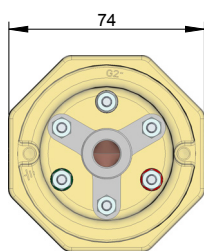
Star connection Y 3x400V
