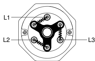
Star connection Y 3x400V
