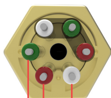
L1 L2 L3 Stjernerkobling
