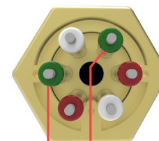
L1 L2 1-fas element
