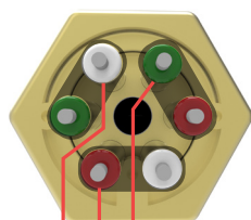
L1 L2 L3 Trekantkobling
