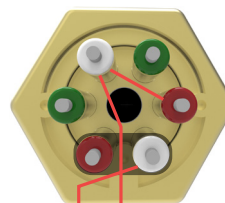
L1 L2 1-fas 2 elementer
