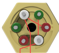
L1 L2 1-fas 3 elementer
