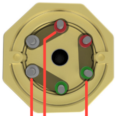
L1 L2 L3 Trekantkobling
