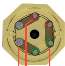
Trekantkobling L1 L2 L3
