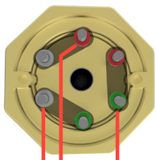
L1 L2 L3 Trekantkobling
