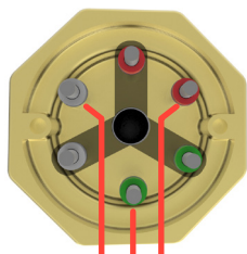
L1 L2 L3 Stjernekobling
