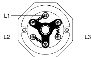
Y-koppling 3x400V
