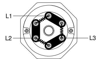
D-koppling 3x400V
